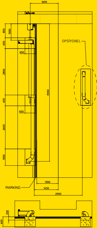
Sol el tipi COMBILOK® SWAP temel betonu ölçüleri
