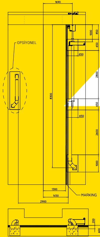
Sağ el tipi COMBILOK® SWAP temel betonu ölçüleri
